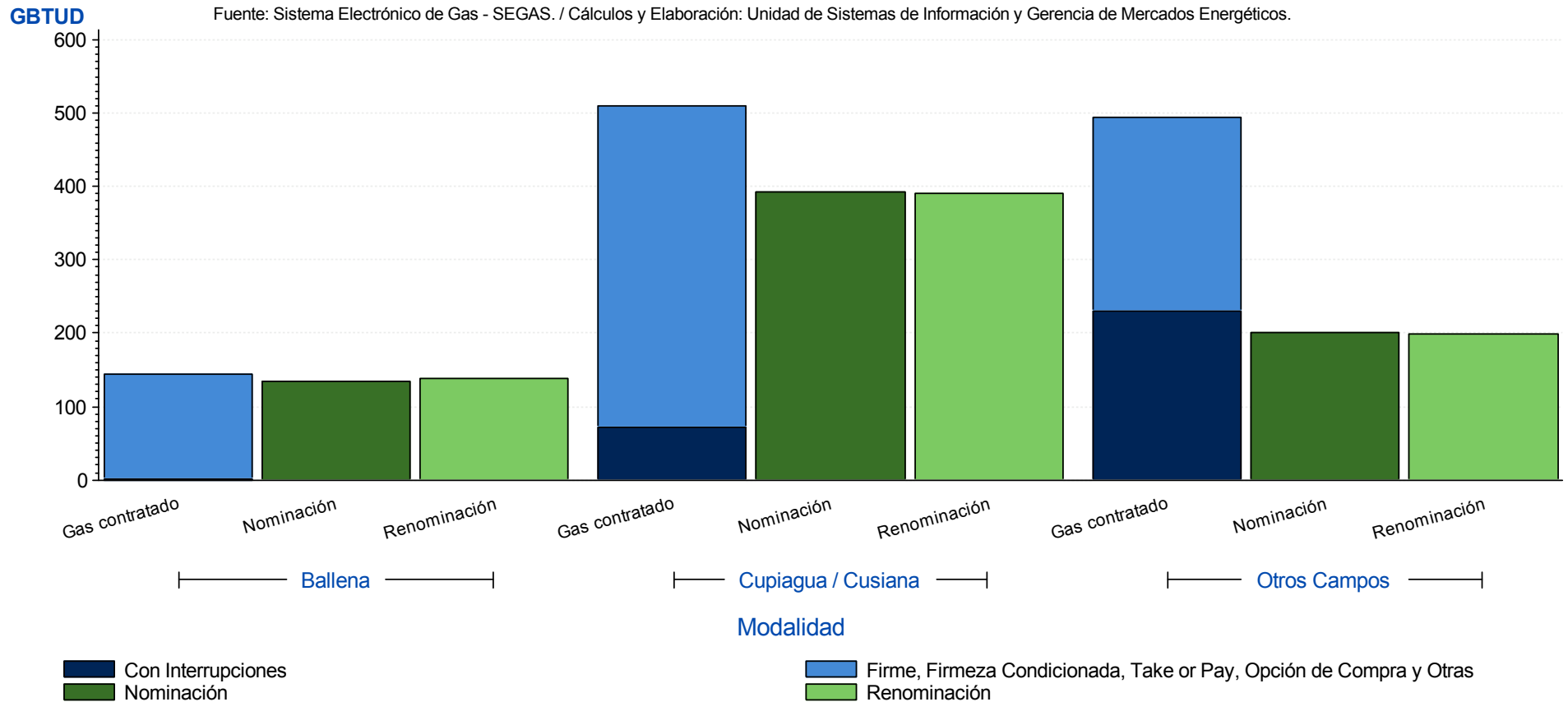
Gráfica 1: Contratación en el Mercado Primario - Suministro de gas. Nominaciones y renominaciones promedio, Octubre de 2018.
