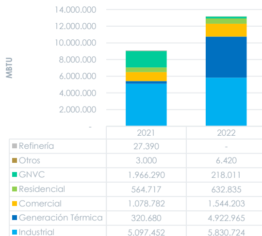
Energía Negociada** MS por Sector Consumo (Neg. Directa) 2022 vs 2021 – Trimestre II
