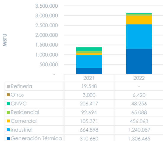
Cantidad agregada Negociada* MS por Sector Consumo (Neg. Directa) 2022 vs 2021 – Trimestre II
